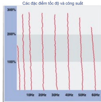
Phương pháp điều khiển vector từ thông tự động đo thông số lớn nhất Momen(%) của mỗi tốc độ (1/5/10/20/30/40/50/60Hz)
