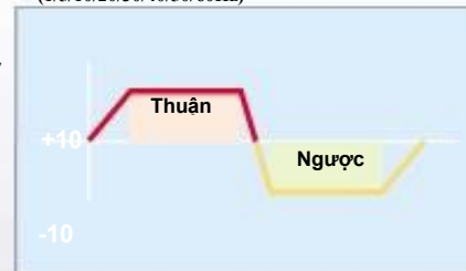
Phương pháp điều khiển vector từ thông tự động đo thông số lớn nhất Momen(%) của mỗi tốc độ (1/5/10/20/30/40/50/60Hz)
